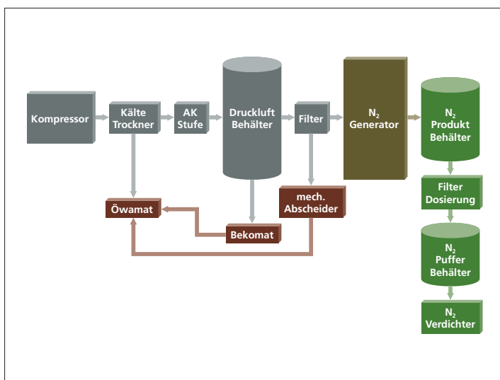
Stickstoffherzeugung aus Druckluft mit PSA-Generator
